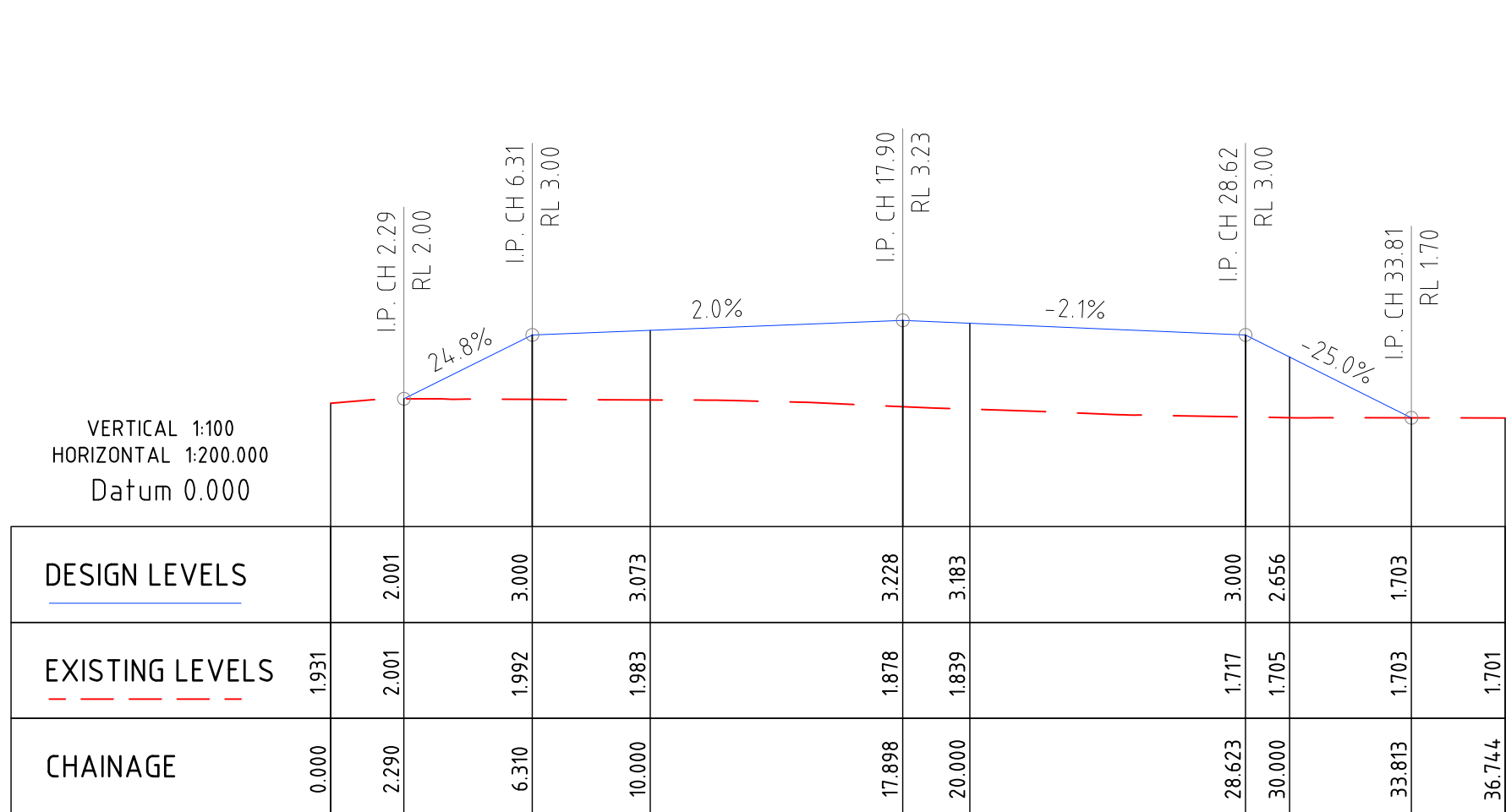
FILL MOUND SECTION B-B
